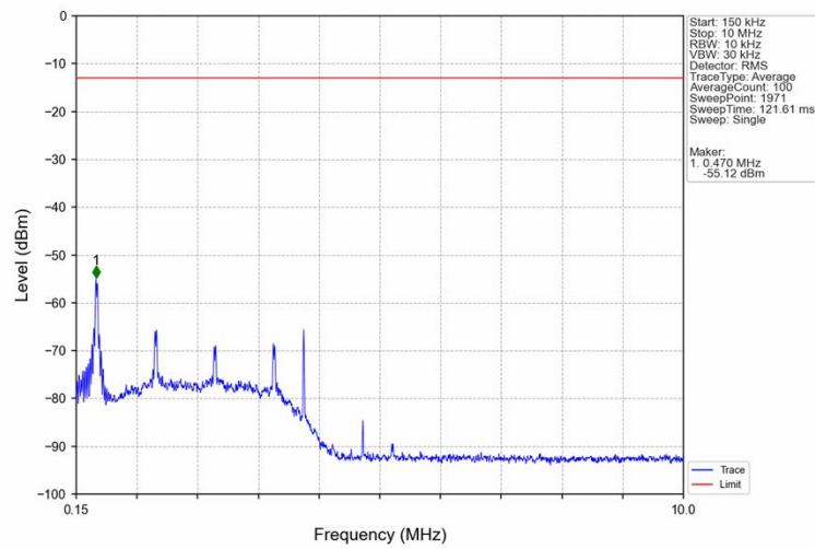
Band5_HSUPA_MCH_836.6MHz_Subtest 1_NTNV
