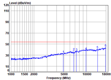
11n_HT(40M)_TX_CH_09_Vertical-Avg
