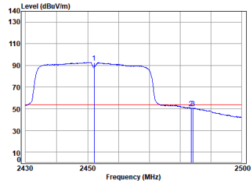
11n_HT(40M)_TX_CH_09_Horizontal-Avg
