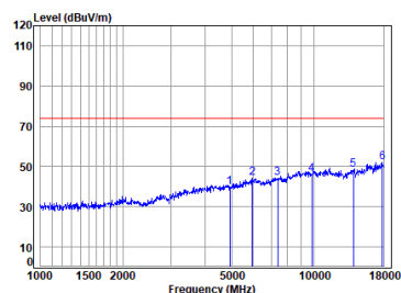
11n_HT(20M)_TX_CH_11_Horizontal-Peak
