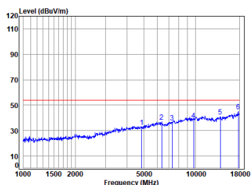
11n_HT(20M)_TX_CH_06_Horizontal-Avg
