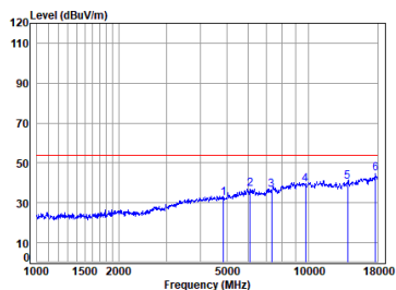
11n_HT(20M)_TX_CH_06_Vertical-Avg
