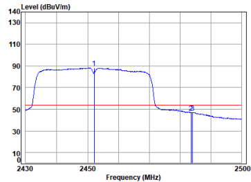
11n_HT(40M)_TX_CH_09_Vertical-Avg
