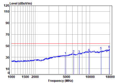
11n_HT(40M)_TX_CH_06_Horizontal-Avg
