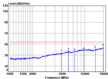
11b_TX_CH_06_Vertical-Avg
