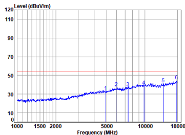
11b_TX_CH_11_Vertical-Avg
