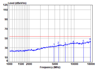
11n_HT(40M)_TX_CH_06_Vertical-Avg
