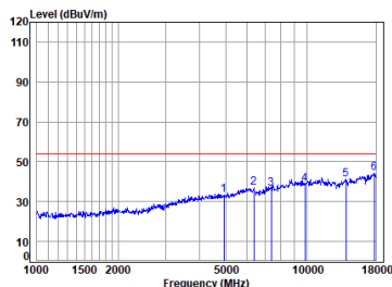
11b_TX_CH_11_Horizontal-Avg
