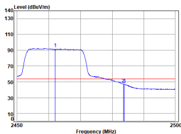
11n_HT(20M)_TX_CH_11_Vertical-Avg
