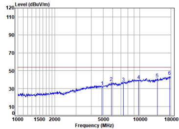
11n_HT(40M)_TX_CH_09_Horizontal-Avg
