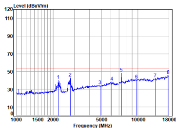
BLE_2M_TX_CH_19_Vertical-Avg
