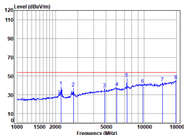
BLE_2M_TX_CH_19_Horizontal-Avg
