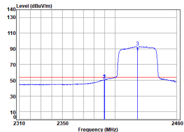
11n_HT(40M)_TX_CH_03_Vertical-Avg
