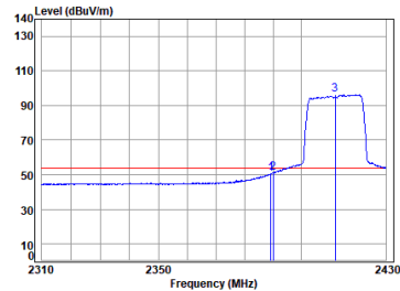
11ax_20M_TX_CH_01_Vertical-Avg
