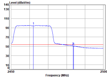
11ax_20M_TX_CH_11_Horizontal-Avg
