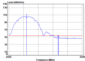
11b_TX_CH_11_Vertical-Avg
