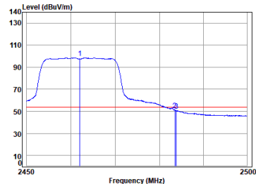
11g_TX_CH_11_Vertical-Avg
