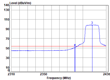
11g_TX_CH_01_Vertical-Avg
