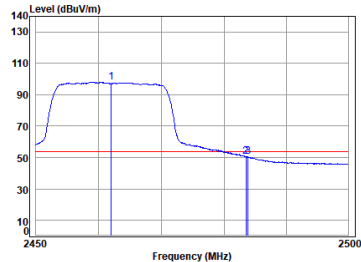
11n_HT(20M)_TX_CH_11_Horizontal-Avg
