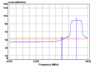
11g_TX_CH_01_Horizontal-Avg
