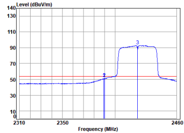
11n_HT(40M)_TX_CH_03_Horizontal-Avg
