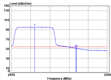
11ax_20M_TX_CH_11_Vertical-Avg
