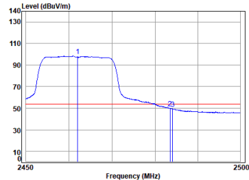
11g_TX_CH_11_Horizontal-Avg
