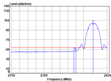
11b_TX_CH_01_Vertical-Avg
