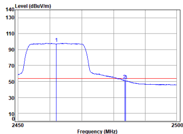
11n_HT(20M)_TX_CH_11_Vertical-Avg
