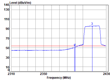
11ax_20M_TX_CH_01_Horizontal-Avg
