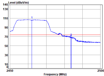
11n_HT(20M)_TX_CH_11_Horizontal-Peak
