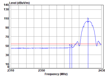
11b_TX_CH_01_Horizontal-Avg
