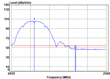
11b_TX_CH_11_Horizontal-Avg
