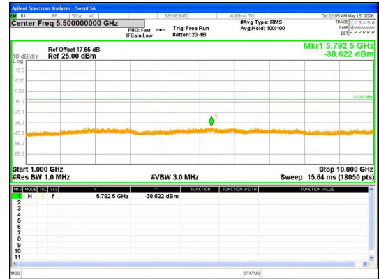
1000.0MHz-10000.0MHz Band 5 5MHz/836.5/Mid 16QAM 1@0
