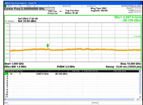
1000.0MHz-10000.0MHz Band 12 5MHz/701.5/Low QPSK 1@0
