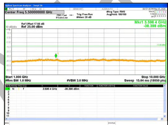
1000.0MHz-10000.0MHz Band 12 5MHz/701.5/Low 16QAM 1@0
