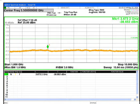
1000.0MHz-10000.0MHz Band 12 5MHz/707.5/Mid QPSK 1@0
