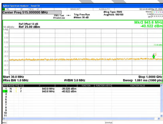
30.0MHz-1000.0MHz Band 12 5MHz/707.5/Mid QPSK 1@0
