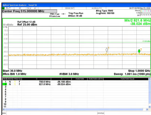
30.0MHz-1000.0MHz Band 12 5MHz/701.5/Low 16QAM 1@0
