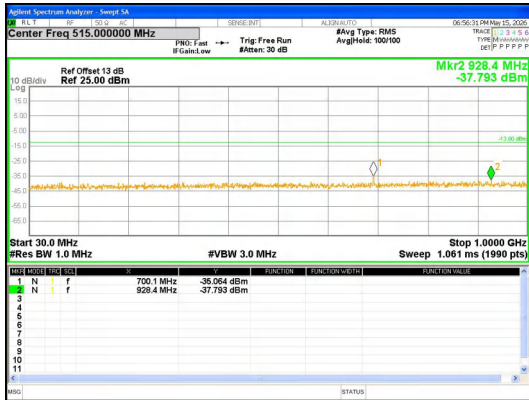
30.0MHz-1000.0MHz Band 12 5MHz/701.5/Low QPSK 1@0
