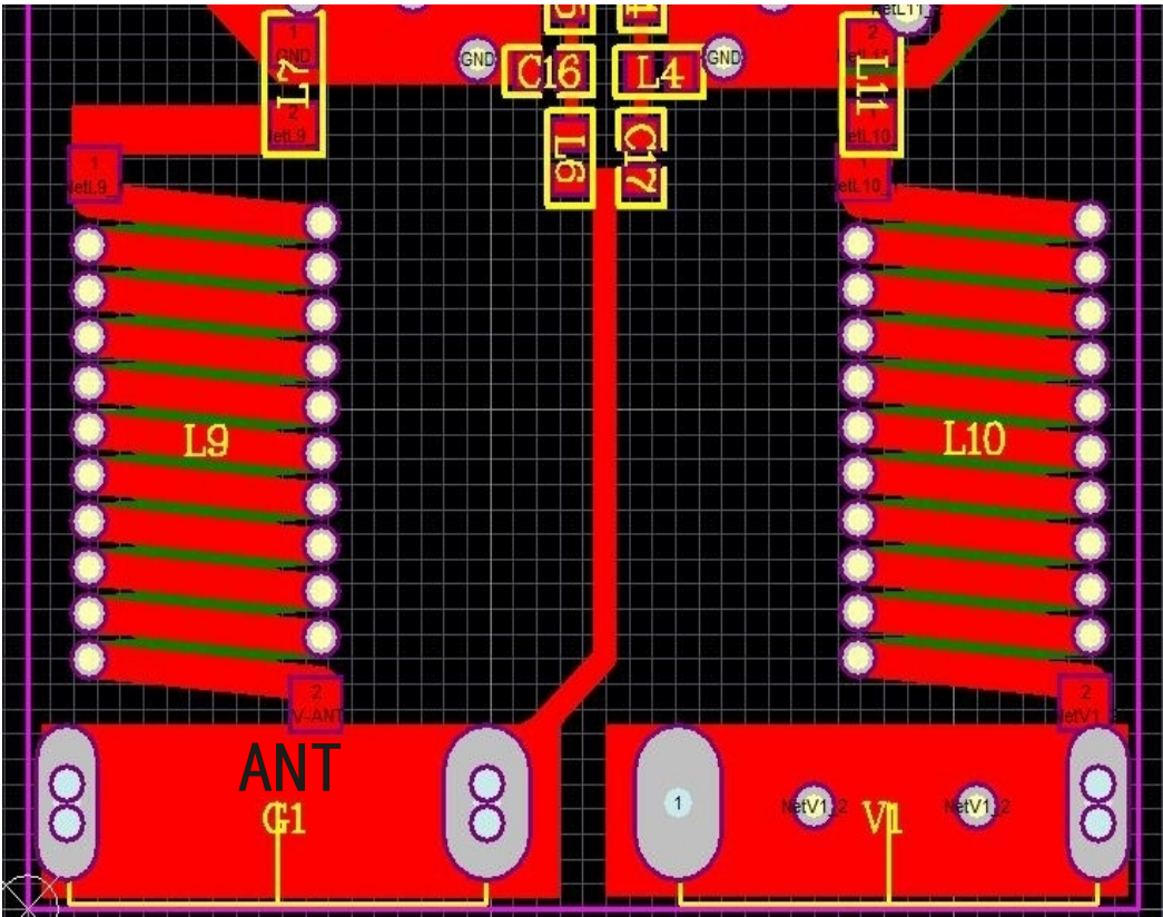
天线图片 Antenna Picture
