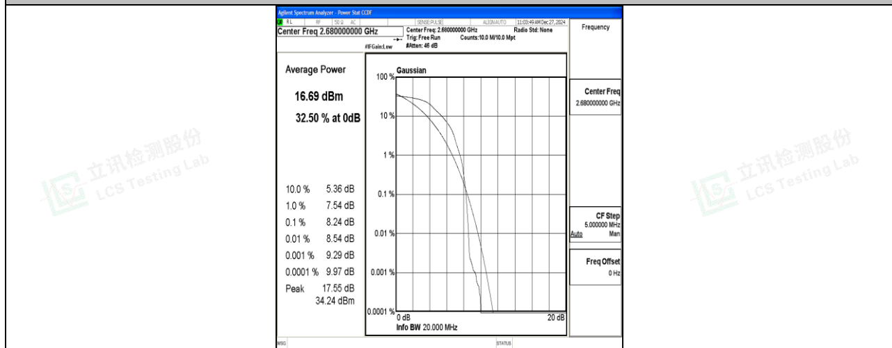
Band41-20MHz-QPSK-41490-1RB#0-PASS
