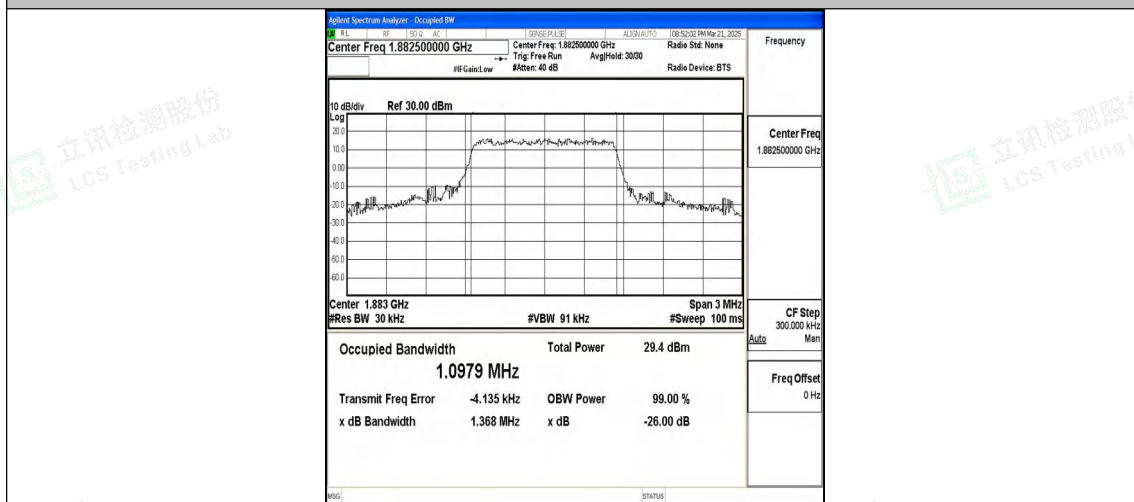
Band25-1.4MHz-QPSK-26365-6RB#0-PASS
