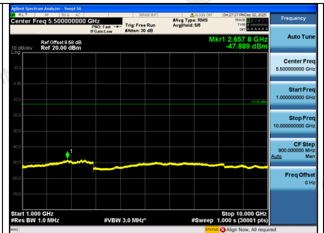
GPRS850-190-5-1000~10000MHz-PASS
