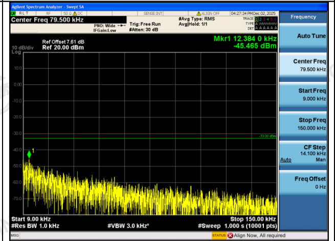
GPRS850-251-5-0.009~0.15MHz-PASS
