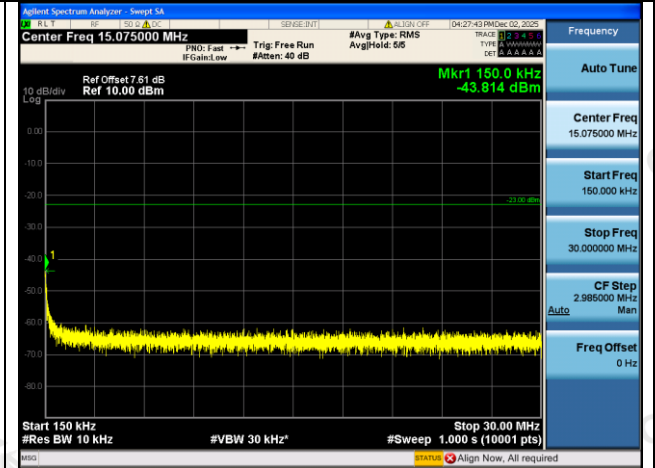
GPRS850-251-5-0.15~30MHz-PASS
