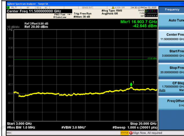
GSM1900-512-0-3000~20000MHz-PASS
