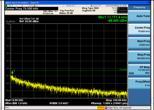
GPRS1900-661-0-0.009~0.15MHz-PASS
