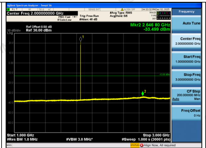
GPRS1900-512-0-1000~3000MHz-PASS
