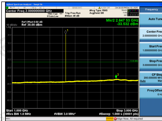
GSM1900-512-0-1000~3000MHz-PASS
