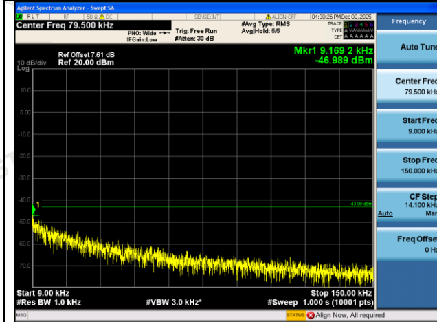
GSM1900-661-0-0.009~0.15MHz-PASS
