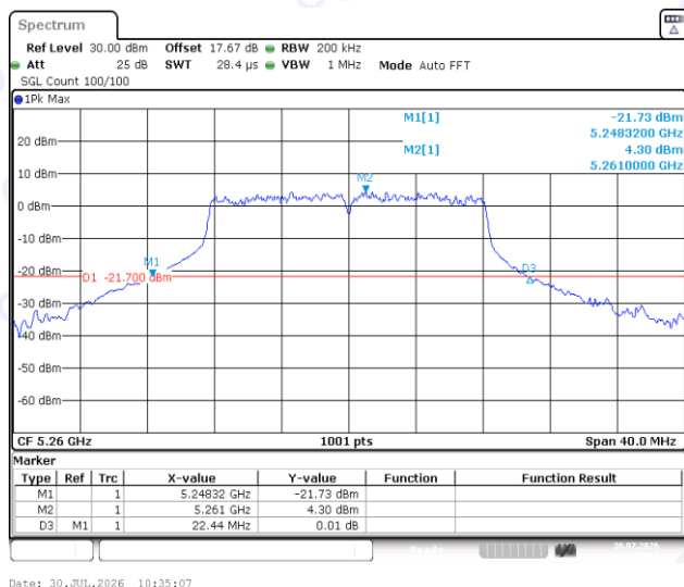
11A-Ant1-5260
