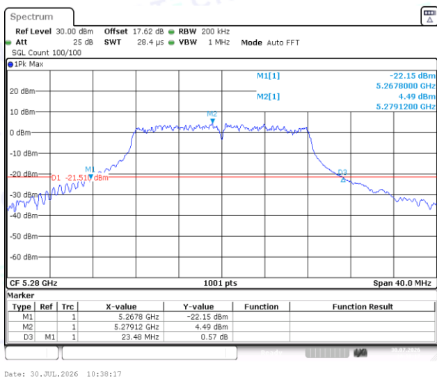
11A-Ant1-5280
