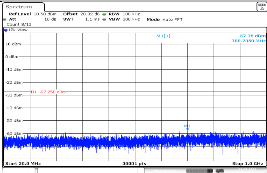
11G-Ant1-2437-30~1000-PASS
