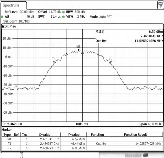
802.11b-Ant1-2462
