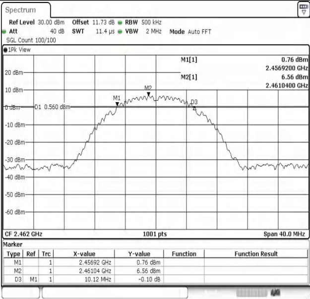
802.11b-Ant1-2462-PASS
