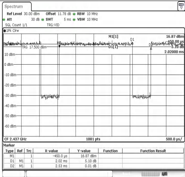
NTNV-802.11g-Ant1-2437
