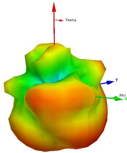
5.5GHz
