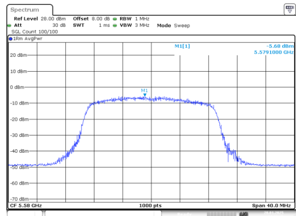
802.11n20_5580MHz
