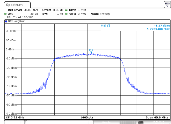
802.11a_5720MHz
