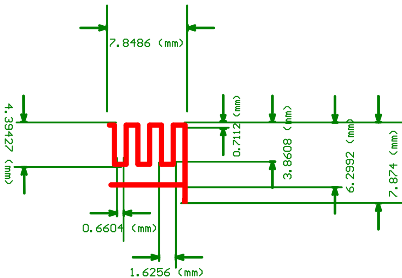
尺寸图
