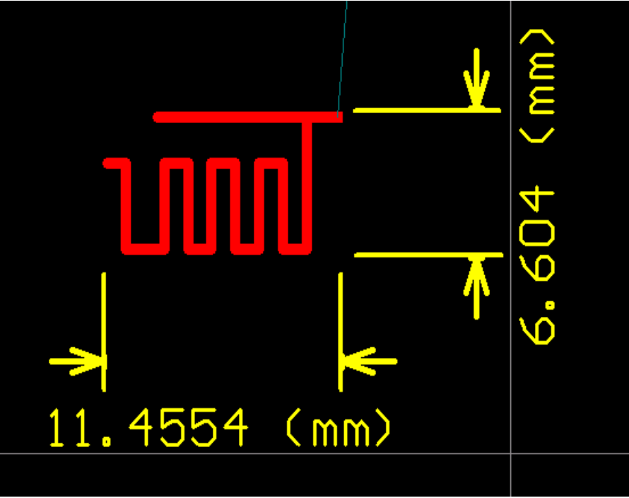
天线尺寸图
