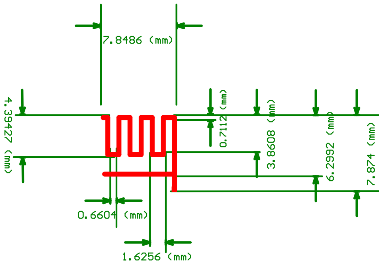
尺寸图
