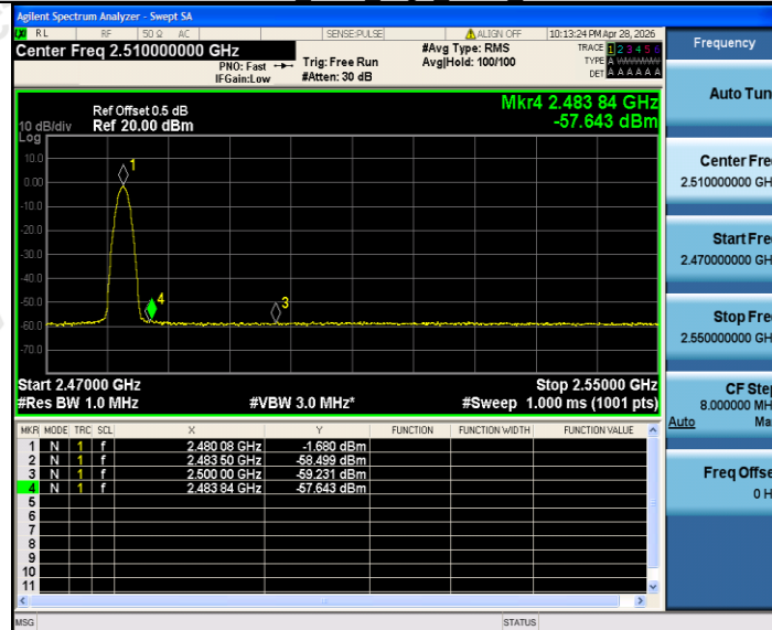
2.4G Ant1 High 2480 AV
