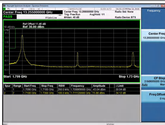
Band66-20MHz-QPSK-132072-1RB#0-PASS
