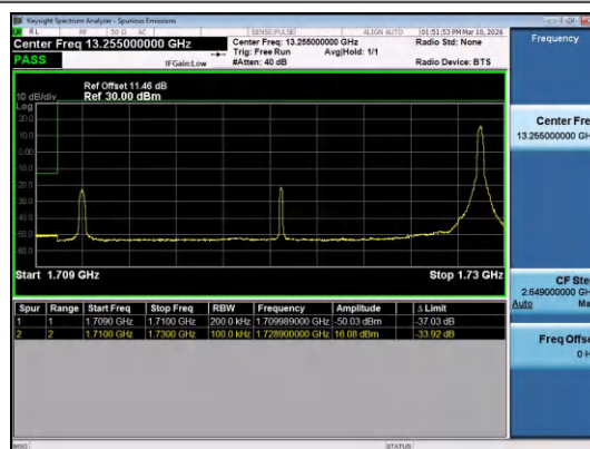
Band66-20MHz-QPSK-132072-1RB#99-PASS
