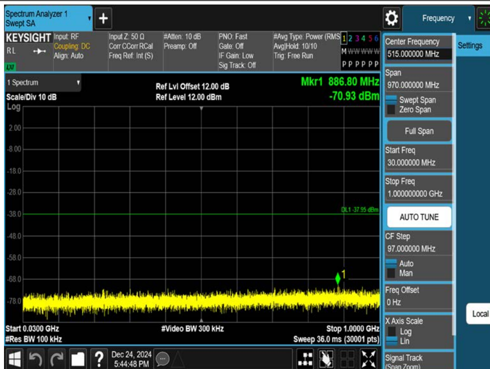
11G-Ant1-2412-30~1000-PASS
