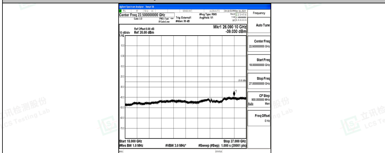
Band38-5MHz-QPSK-38000-25RB#0-18000~27000-PASS
