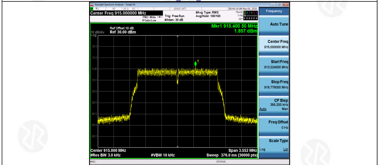
2M Ant1_915
