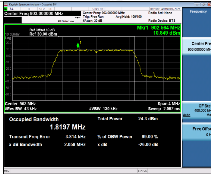
2M Ant1 903
