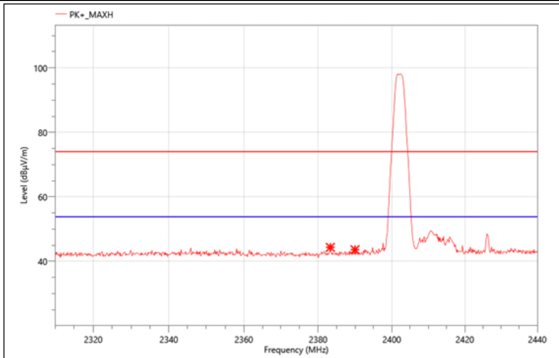
BLE-1M 2402
