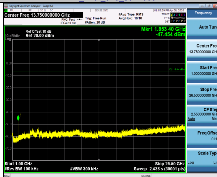
4M_Ant1_926_1000~26500
