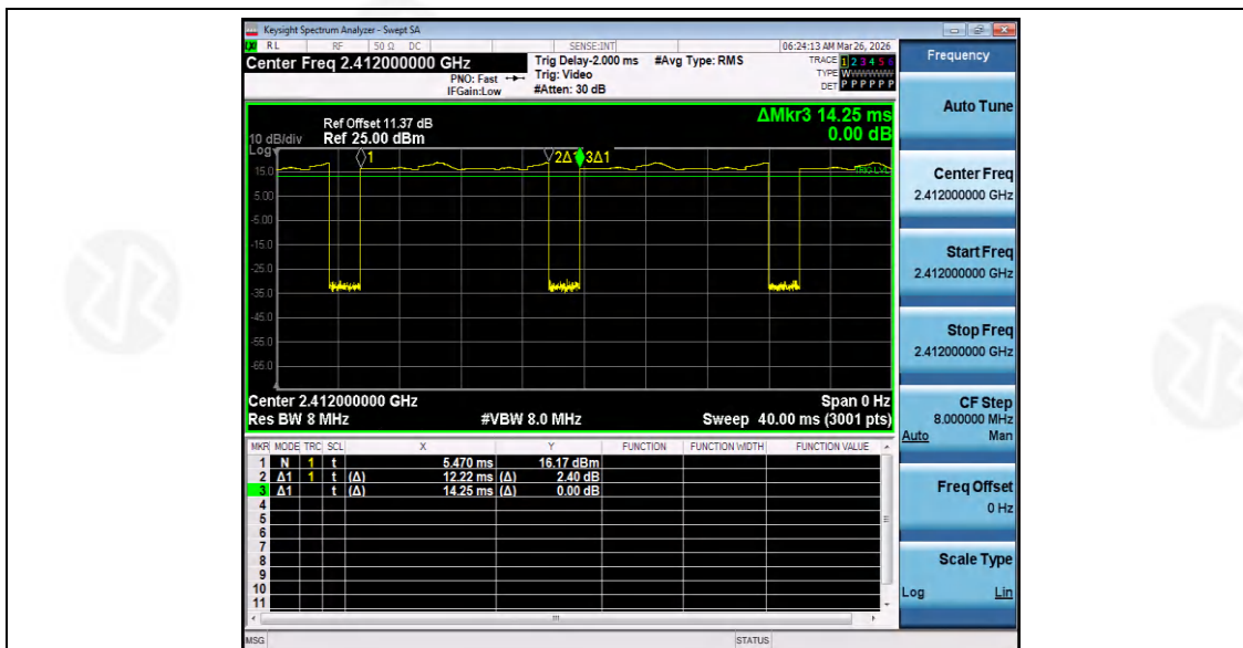
11B_Ant1_2412
