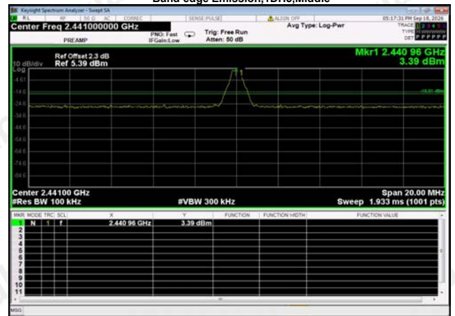
Band edge Emission,1DH5,Middle
