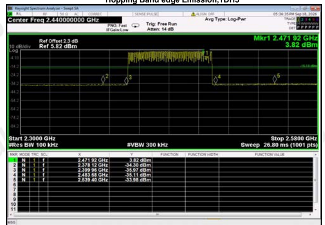
Hopping Band edge Emission,1DH5
