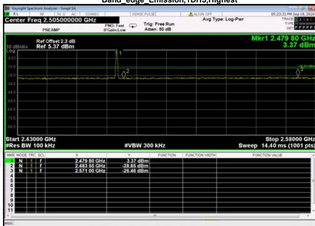
Band edge Emission,1DH5,Highest
