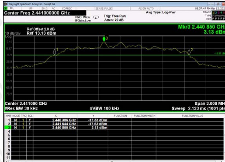
CH39
