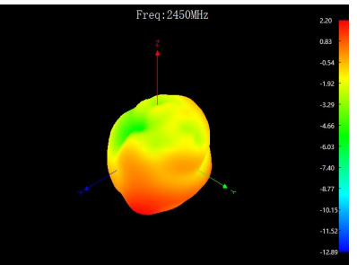
YZX face @2450MHz
