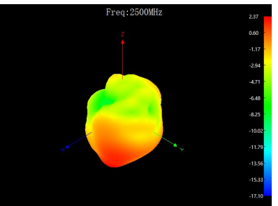
YZX face @2500MHz
