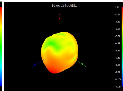
YZX face @2400MHz
