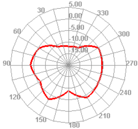
2480.000MHz E1
