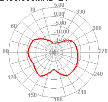
2430.000MHz E1
