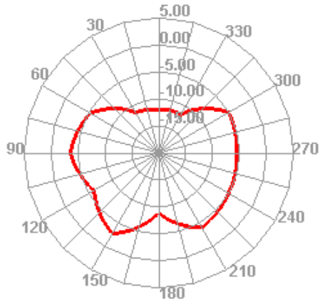
2490.000MHz
