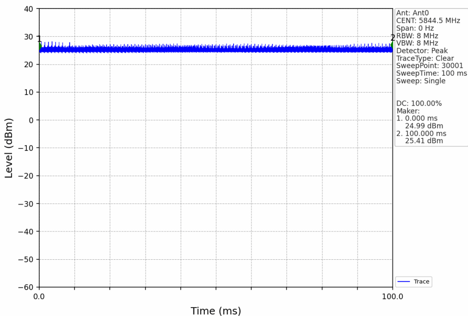
10M_HCH_5844.5MHz_Ant0_NTNV
