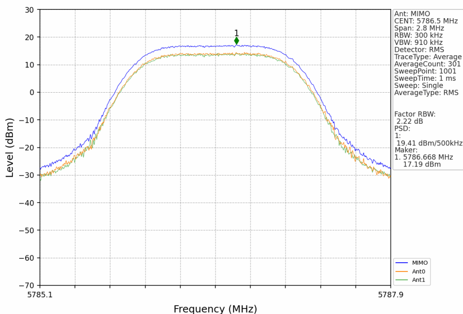
1.4M_MCH_5786.5MHz_MIMO_NTNV
