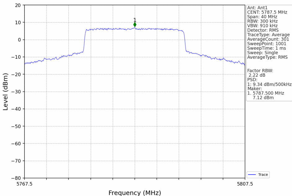
20M_MCH_5787.5MHz_MIMO_NTNV
