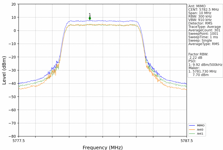
5M_MCH_5782.5MHz_MIMO_NTNV
