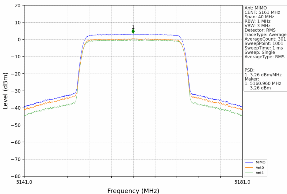
20M_LCH_5161MHz_MIMO_NTNV
