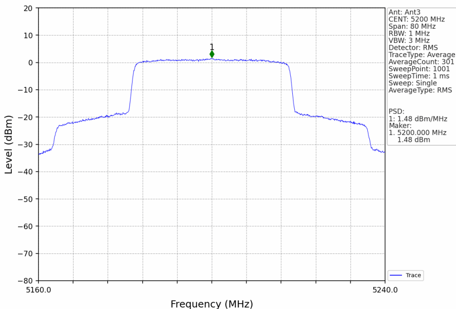
40M_MCH_5200MHz_MIMO_NTNV
