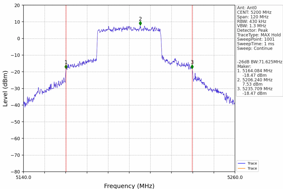
40M_MCH_5200MHz_Ant0_NTNV
