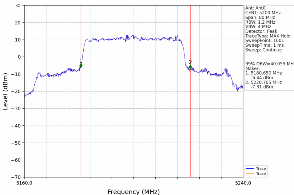
40M_MCH_5200MHz_Ant0_NTNV
