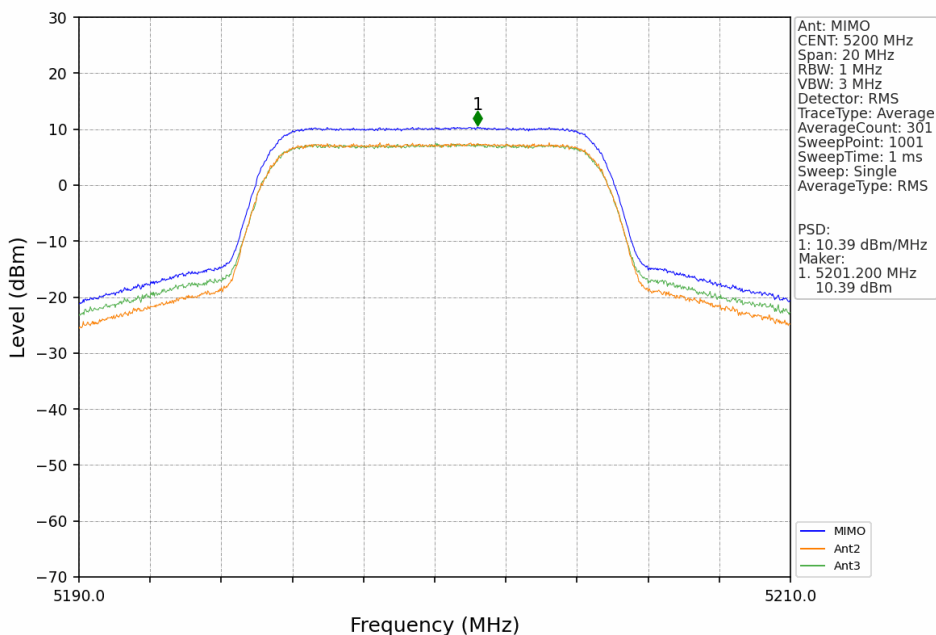
10M_MCH_5200MHz_MIMO_NTNV
