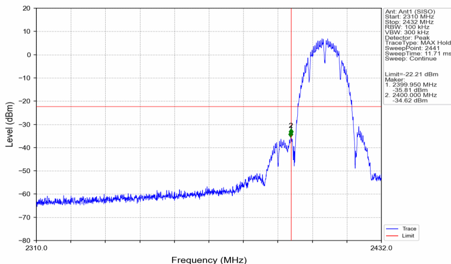
802.11b_LCH_2412MHz_Ant1 (SISO)_NTNV
