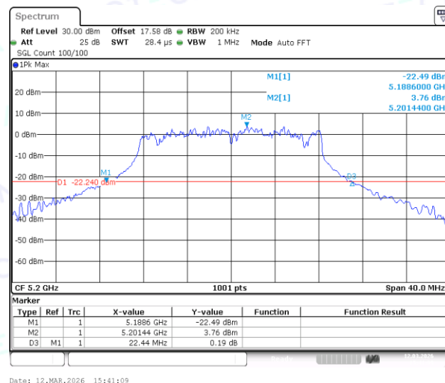
11A-Ant1-5200
