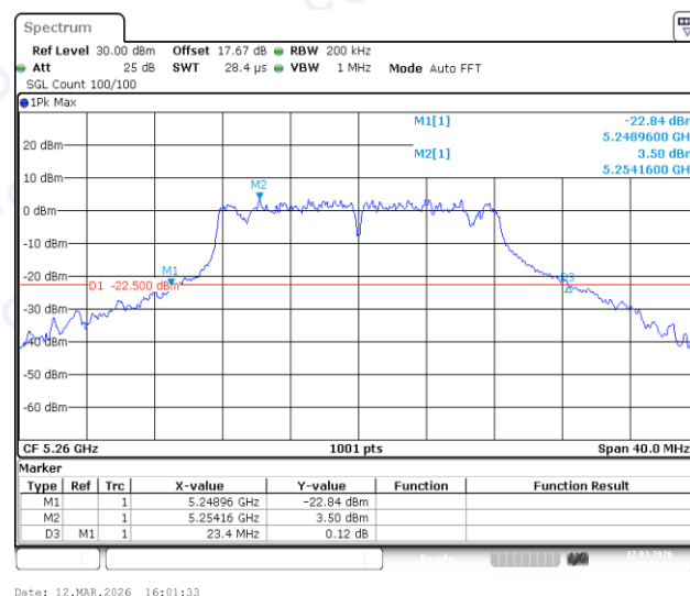
11A-Ant1-5260
