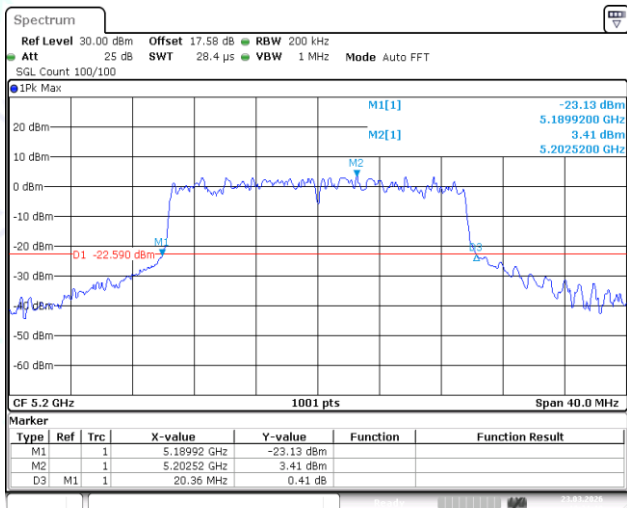
11AX20SISO-Ant1-5200
