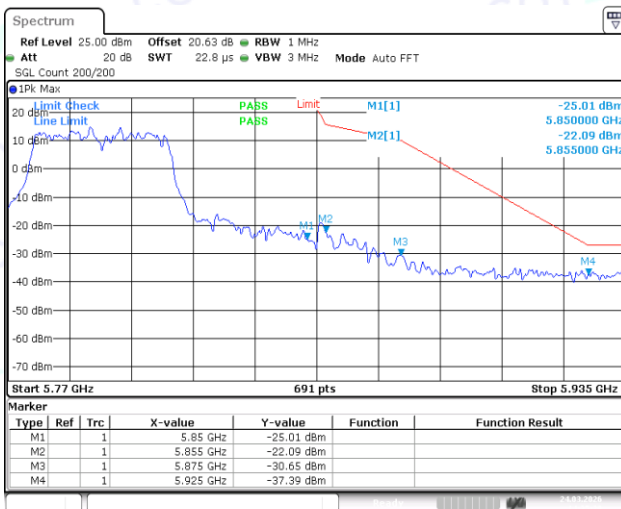
11N40SISO-Ant1-5755-PASS
