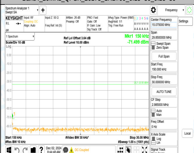
Band4 20MHz QPSK 20175 1RB#99 1000~3000 1000~3000
