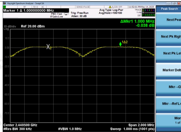
GFSK
