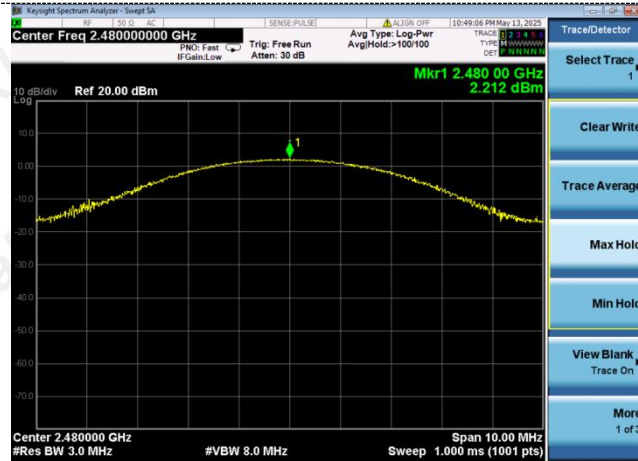
GFSK(CH78)
