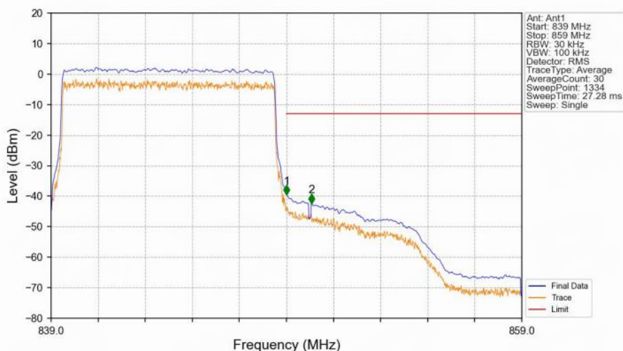
Band5_10MHz_QPSK_HCH_844MHz_RB_50_0_NTNV
