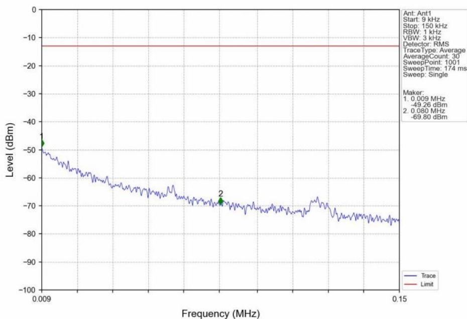
Band5 10MHz 16QAM LCH 829MHz RB 1 0 NTNV
