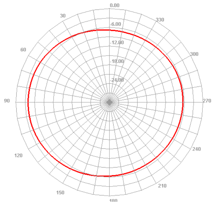
830.000MHz E2
