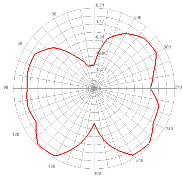
830.000MHz E2
