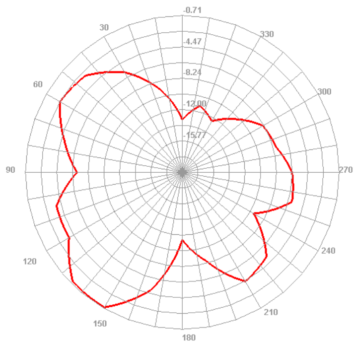
830.000MHz E1
