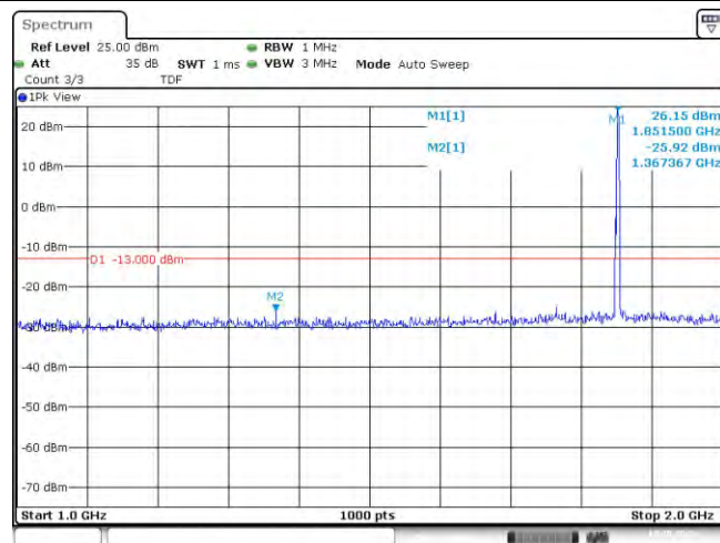
Band2-1.4MHz-QPSK-18607-6RB#0-Range2:1000~2000MHz
