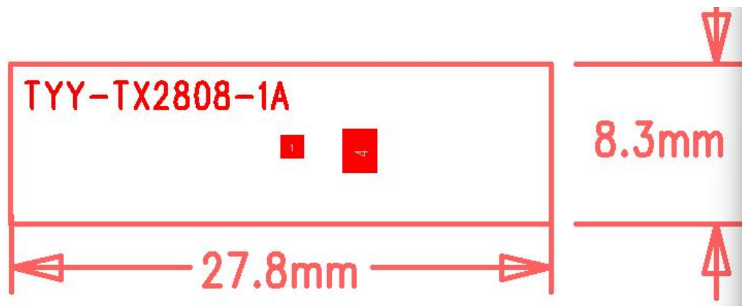
图 2 TYY-TX2808-1A WIFI 天线成品(线长 55mm 带 3 代端子)
