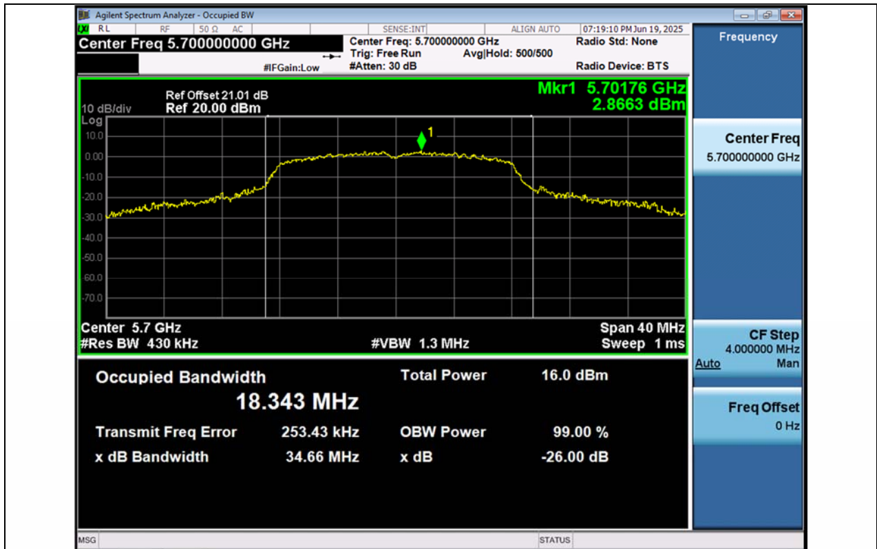
11A-Ant1-5700
