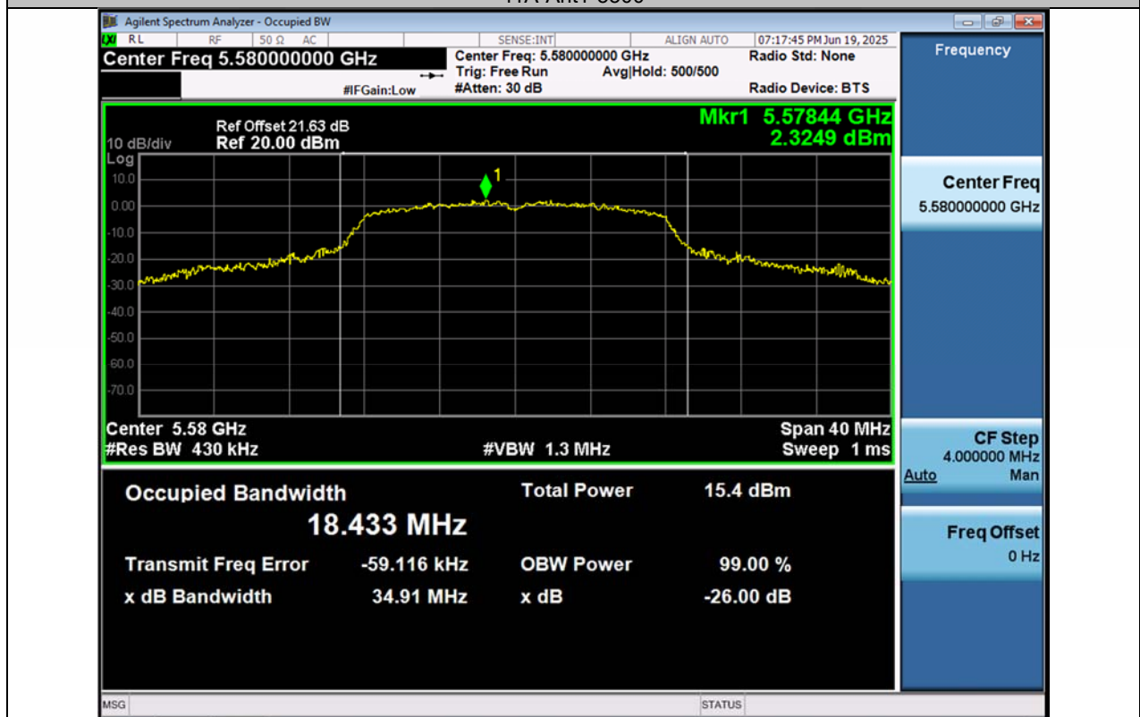
11A-Ant1-5580
