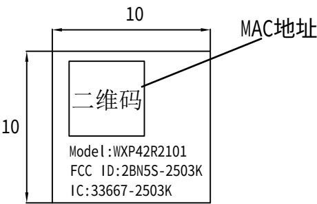
印制板标签
