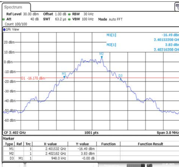
DH5-Ant1-2402
