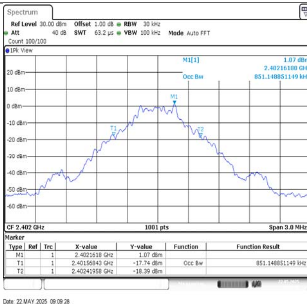
DH5-Ant1-2402
