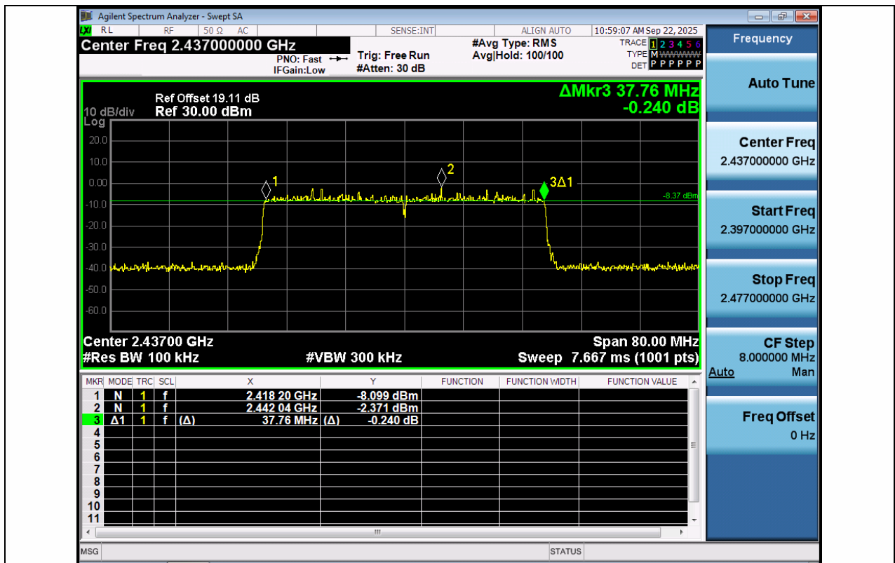
11AX40MIMO-Ant1-2437-PASS
