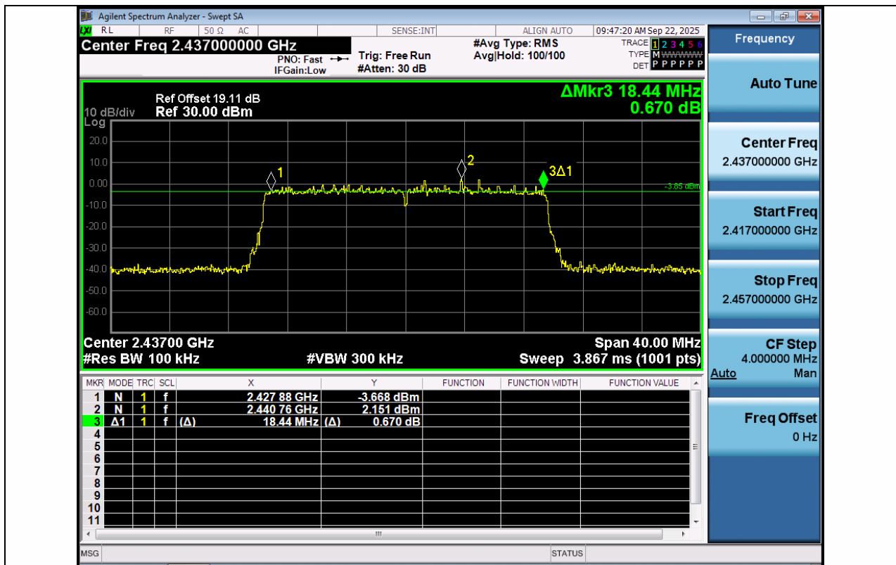
11AX20MIMO-Ant1-2437-PASS
