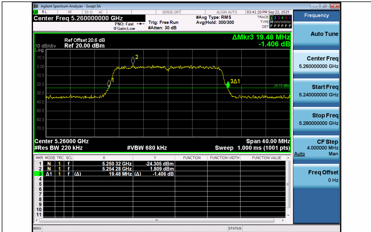
11N20MIMO-Ant1-5260
