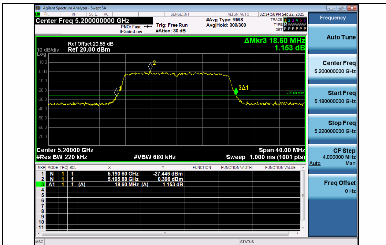
11A-Ant1-5200
