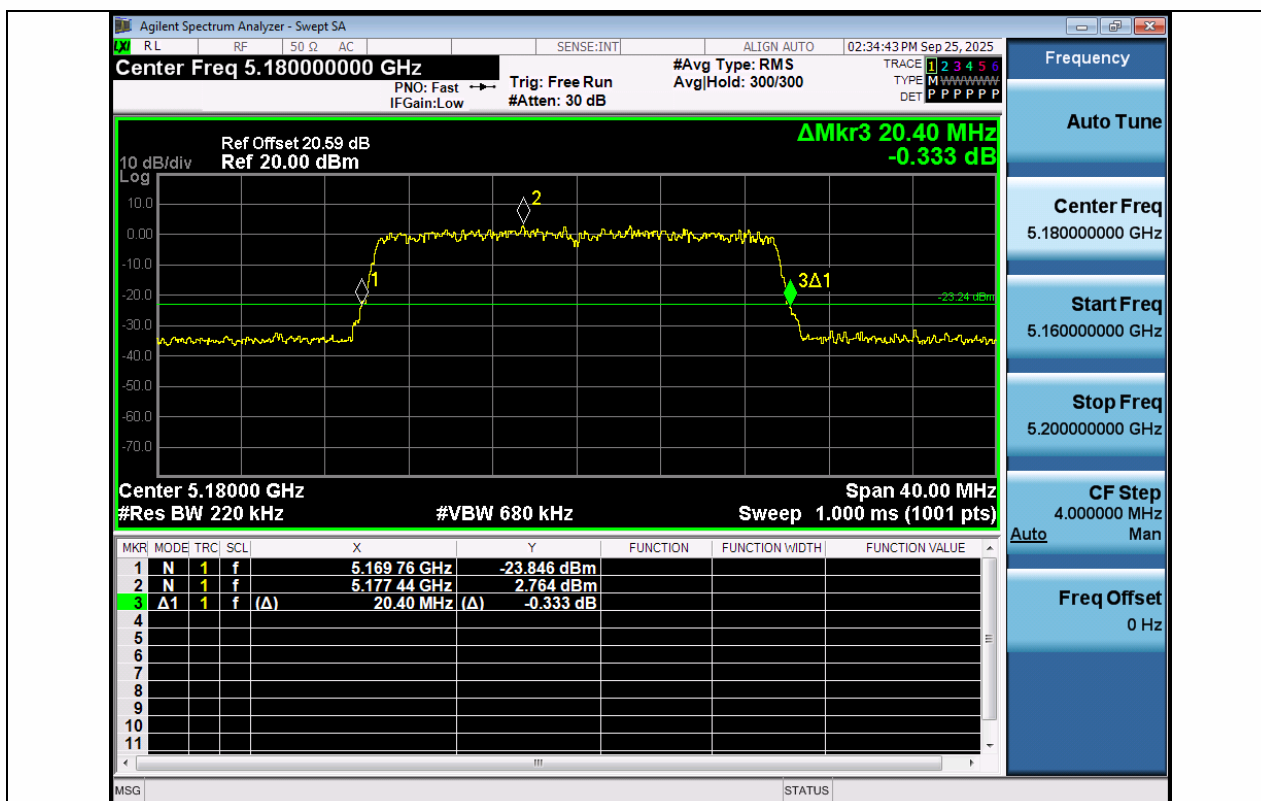
11AX20MIMO-Ant1-5180
