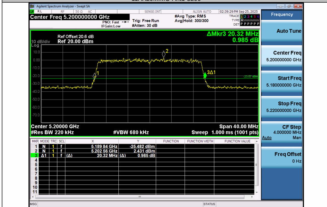
11AX20MIMO-Ant2-5200
