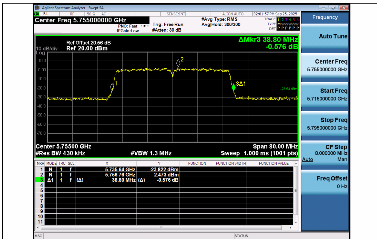
11AC40MIMO-Ant1-5755
