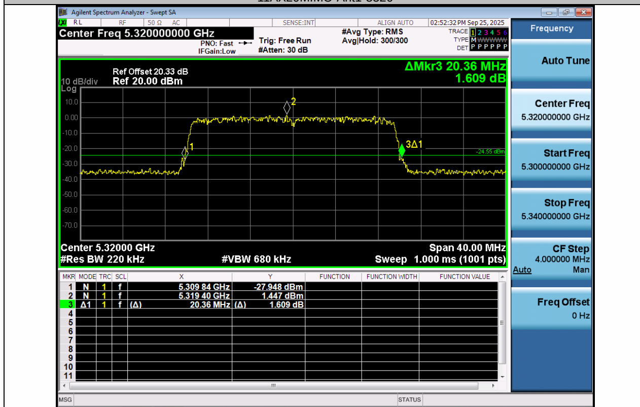
11AX20MIMO-Ant2-5320
