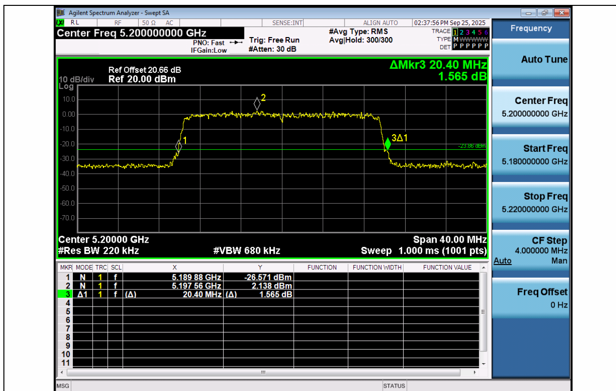
11AX20MIMO-Ant1-5200
