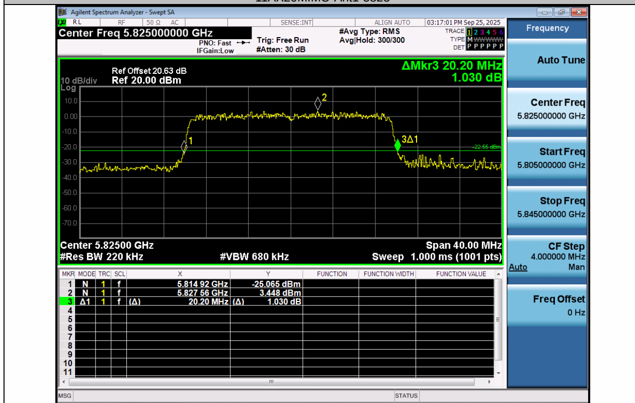
11AX20MIMO-Ant2-5825
