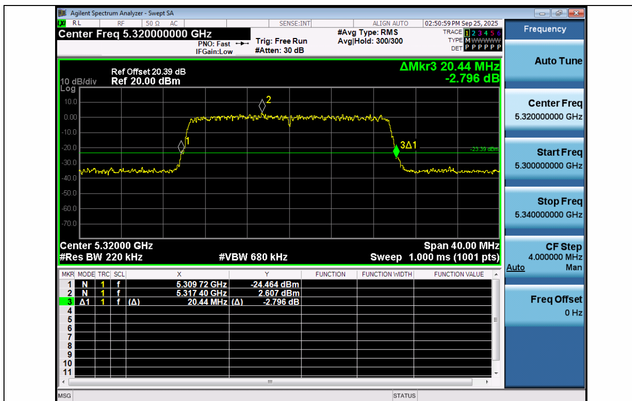
11AX20MIMO-Ant1-5320
