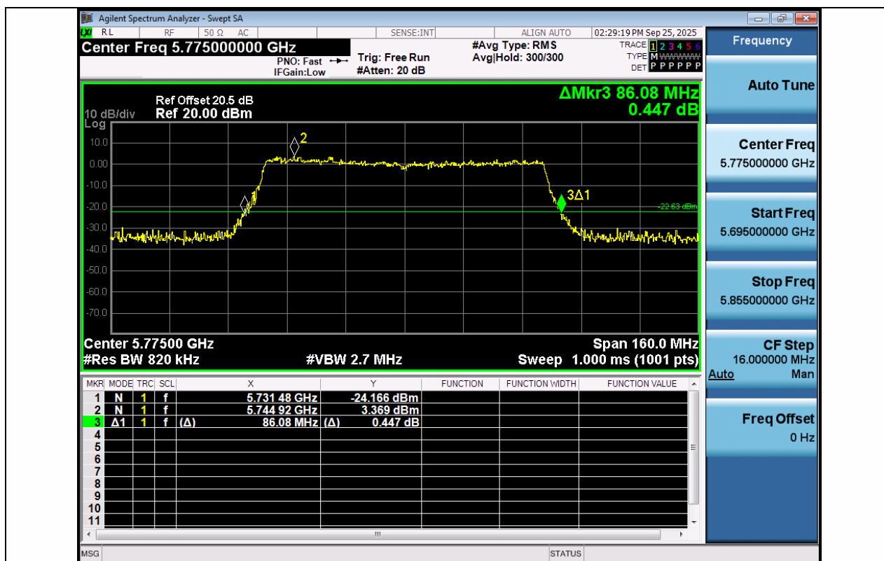
11AC80MIMO-Ant1-5775
