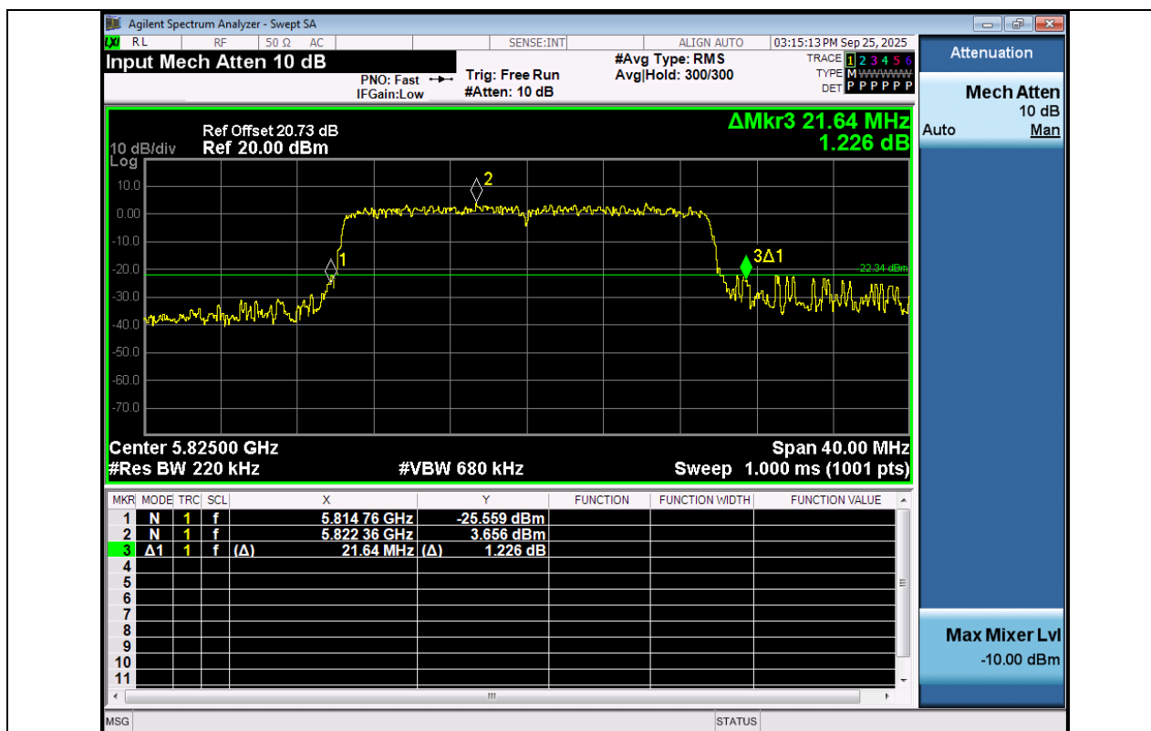
11AX20MIMO-Ant1-5825
