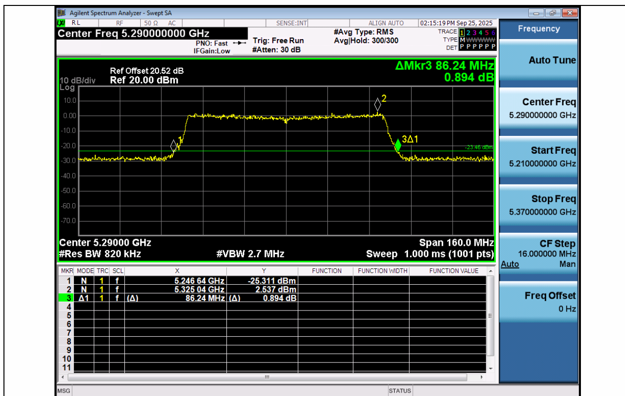
11AC80MIMO-Ant1-5290
